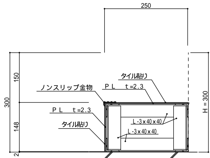
断面図 S = 1 : 5
